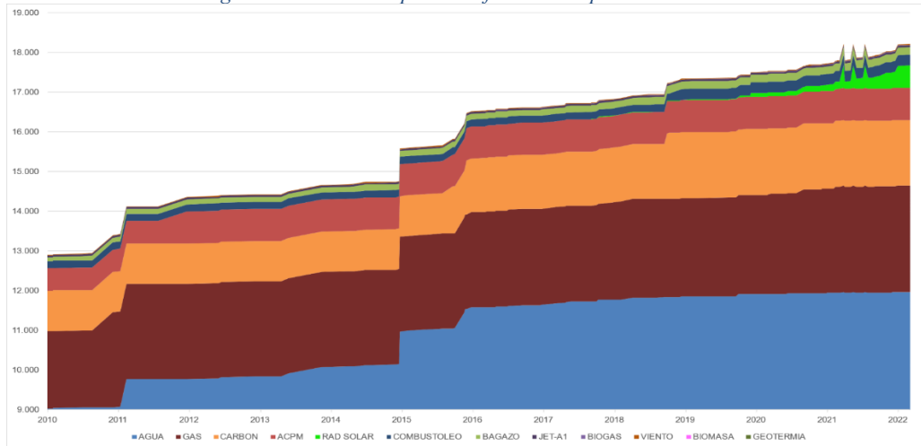
Figura 3. Evolución capacidad efectiva neta por combustible.
